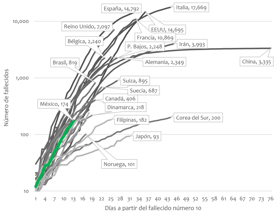
Evolución de fallecidos por país
